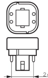
G24q2
